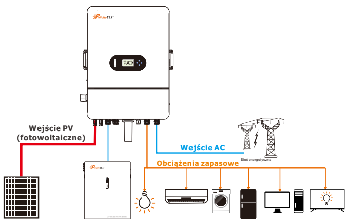
Rysunek 2.1-1 Schemat blokowy systemu falownika słonecznego hybrydowego
