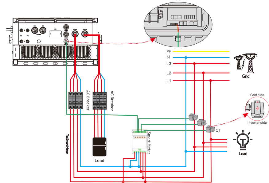
Rysunek 4.4-2 Połączenie inteligentnego licznika
