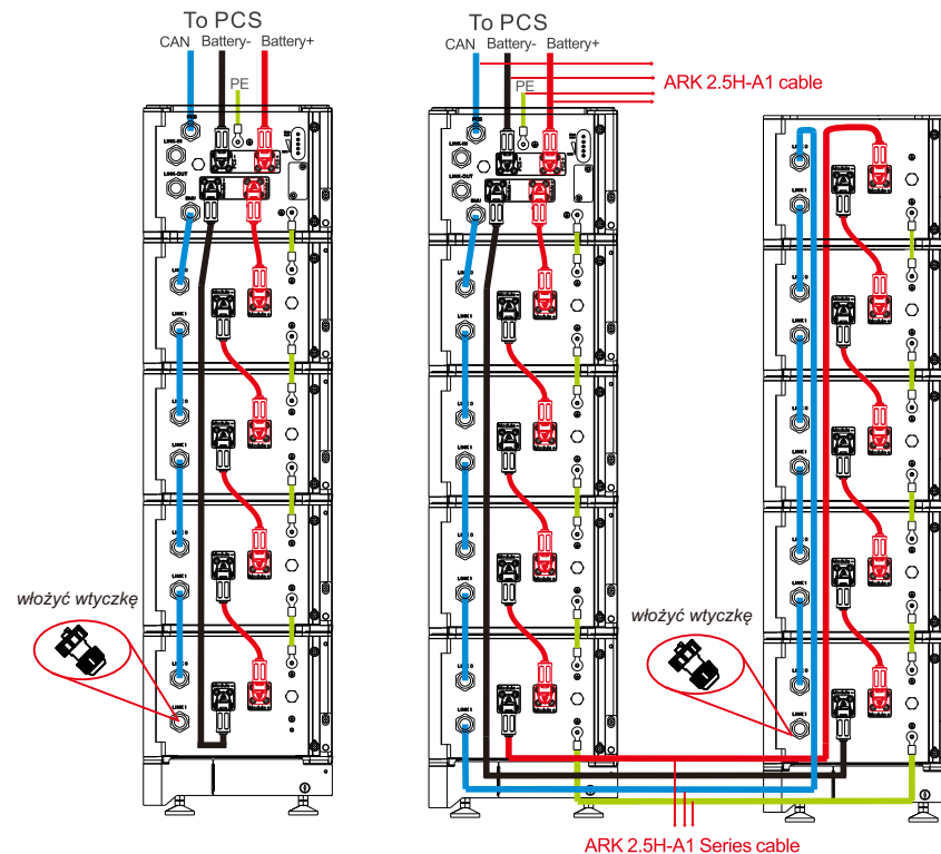
Rys. 4.9: Instalacja pojedynczej linii
