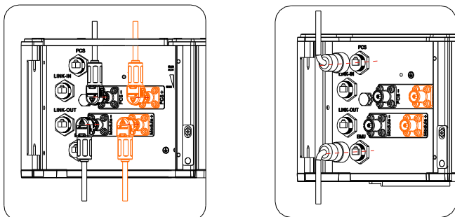
Rys. 4.11: Schemat połączeń elektrycznych HVC60050-A1
