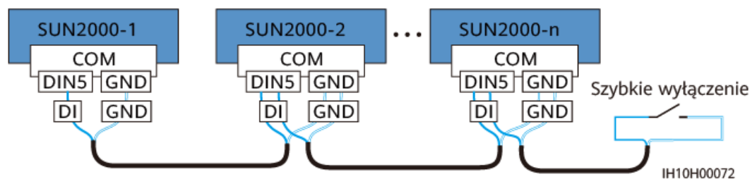
Rysunek 5-32 Podłączanie falowników połączonych kaskadowo do przełącznika szybkiego wyłączania
