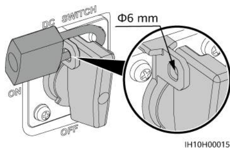
Rysunek 4-9 Zakładanie kłódki zabezpieczającej przełącznik DC
