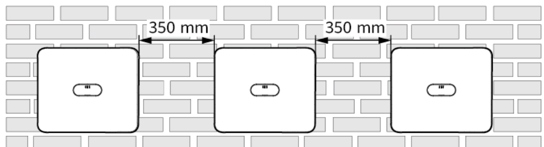
Rysunek 4-3 Montaż w układzie poziomym (zalecany)
