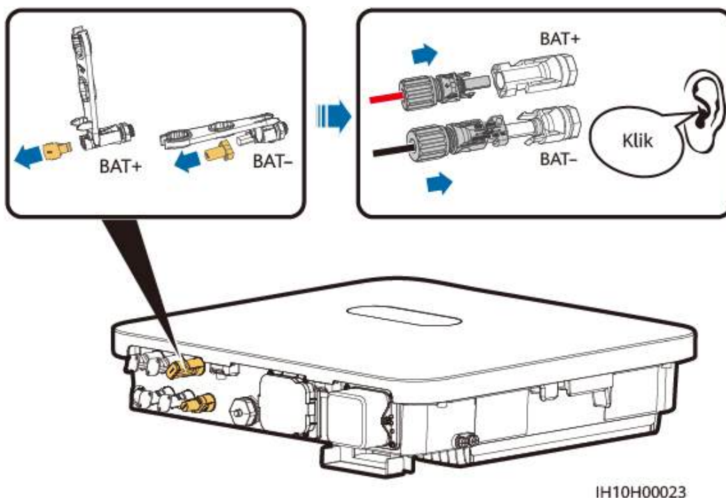
Rysunek 5-12 Podłączanie przewodów akumulatora
