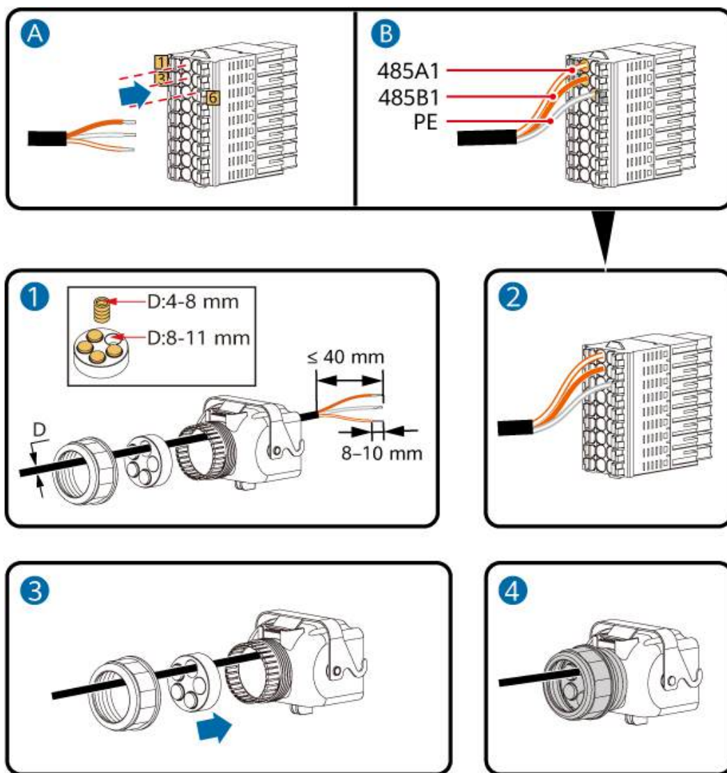
Rysunek 5-19 Instalacja kabla
