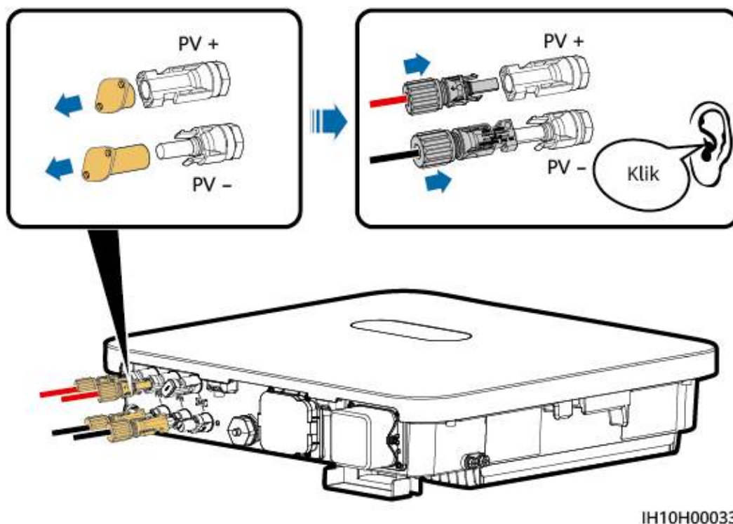
Rysunek 5-10 Podłączanie wejściowych kabli zasilania DC
