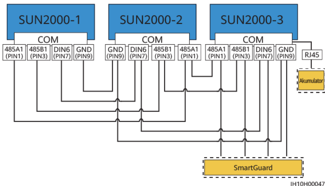
Rysunek 5-17 Połączenie sieciowe z użyciem modułu SmartGuard (części obrysowane przerywaną linią są opcjonalne)
