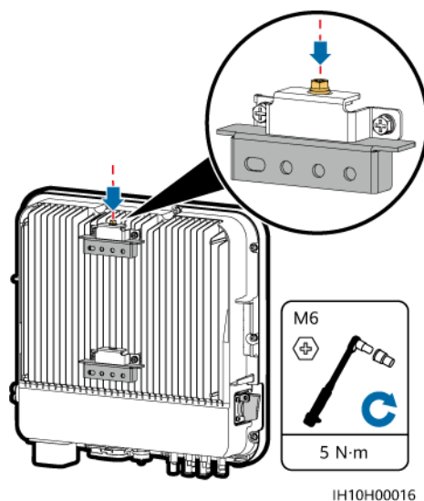
Rysunek 4-10 Montaż falownika
