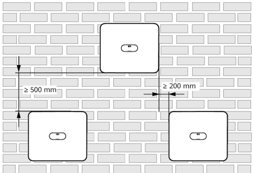
Rysunek 4-4 Montaż w układzie trójkątnym (zalecany)
