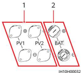
Rysunek 5-7 Zaciski
