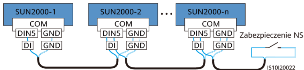
Rysunek 5-38 Podłączanie falowników kaskadowych do przełącznika zabezpieczenia NS
