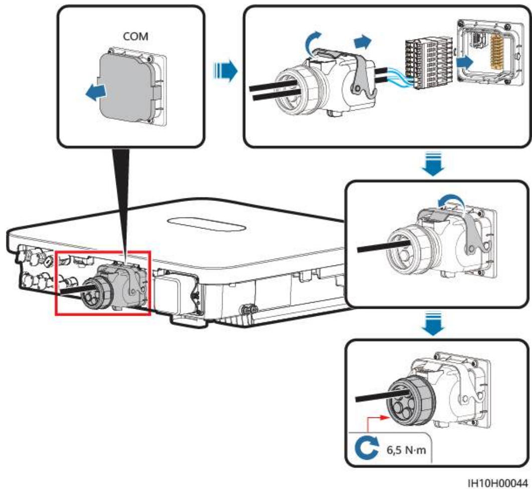
Rysunek 5-40 Zabezpieczanie złącza kabla sygnałowego
