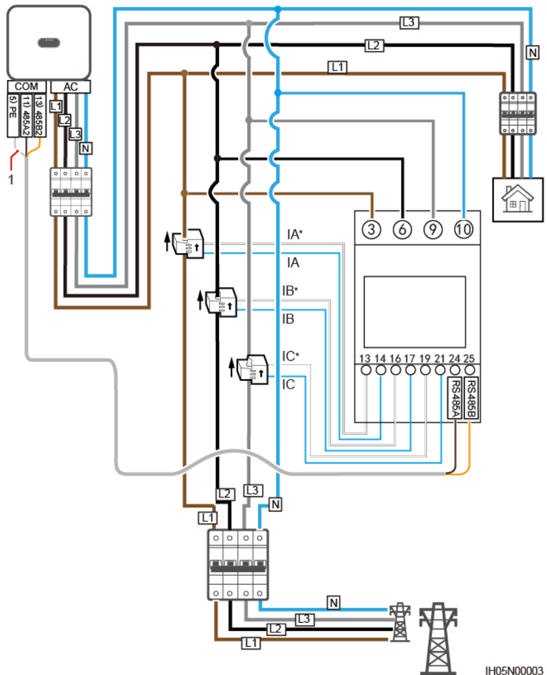
Rysunek 5-23 Połączenie trójfazowe, czterożyłowe (połączenie sieciowe Smart Dongle)
