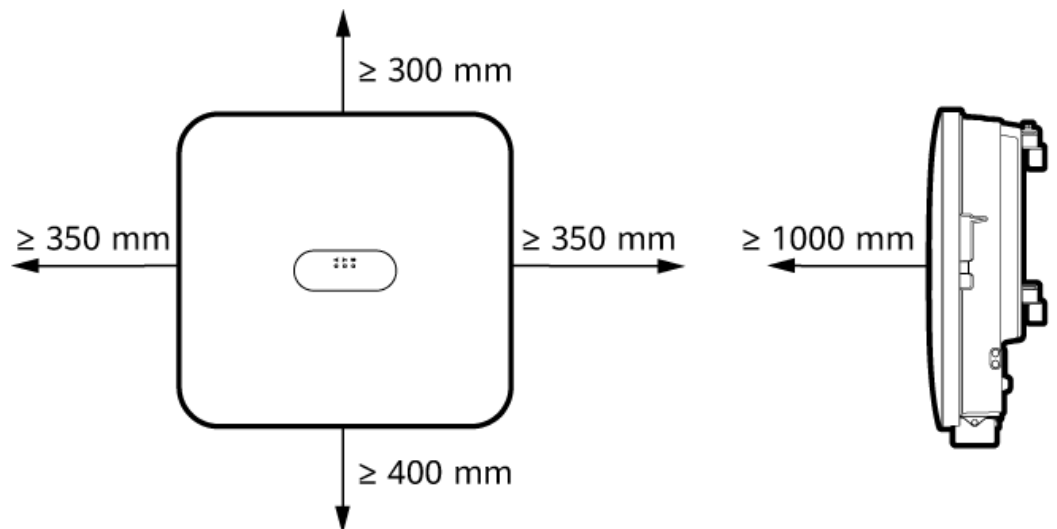
Rysunek 4-2 Odstępy
