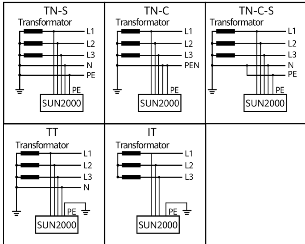
Rysunek 2-6 Obsługiwane sieci elektryczne
