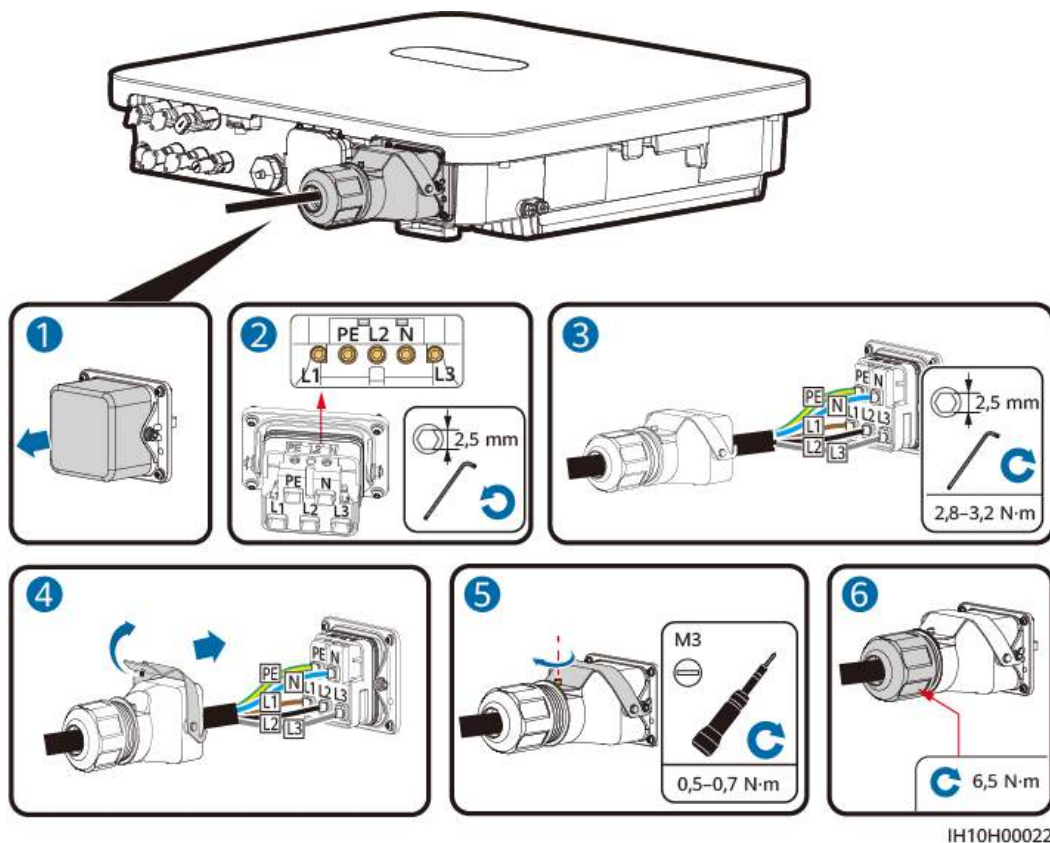
Rysunek 5-5 Zabezpieczanie złącza AC
